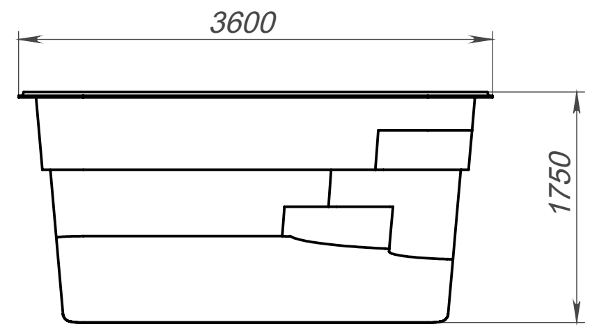
Вид 4-4
