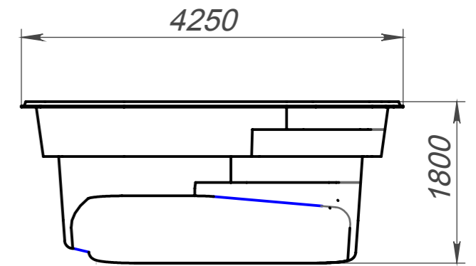
Вид 4-4
