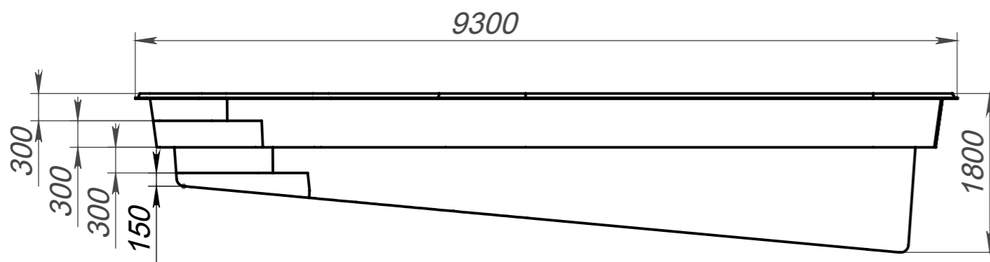
Вид 2-2
